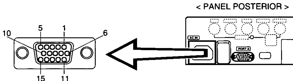
Asignación de los contactos de miniconector D-sub de 15 contactos
