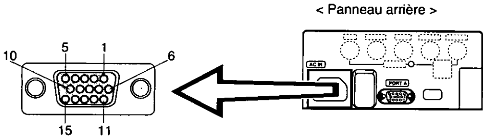
Affectation des broches de la miniprises à 15 broches D-Sub
